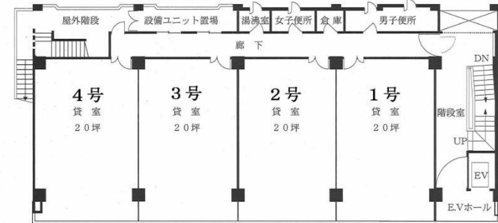
2階～4階平面図
