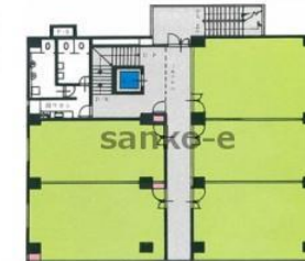
2階～6階平面図
